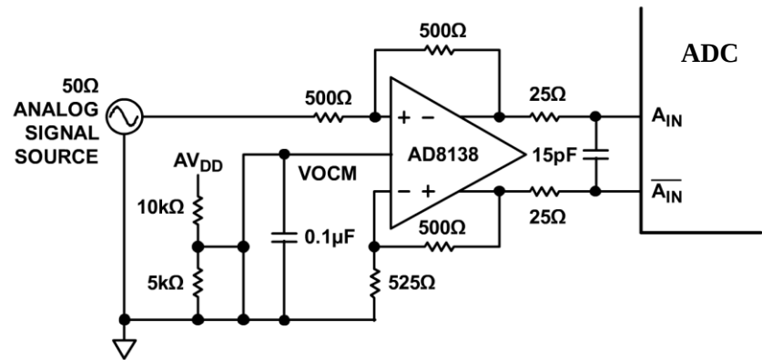
图 8 AD8138 驱动 ADC
