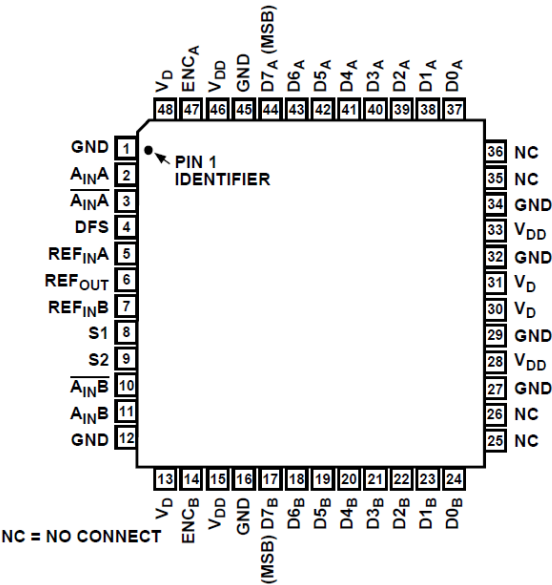
图 2 管脚分布
